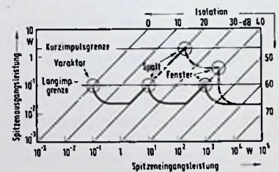
Bild 11. Charakteristik eines passiven TRL
