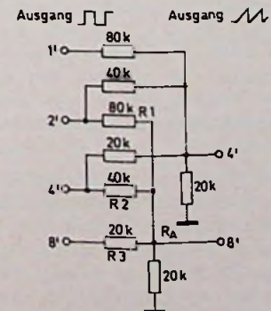
Bild 4. Beschaltung der integrierten Schaltung SAH 220 als Treppenspannungs-/Sägezahn-Generator
