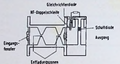
Bild 7. Querschnitt durch einen Gas-Dioden-Limiter (GDL)
