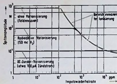
Bild 6. Einfluß der Pulsiederholrate auf die Spitzenamplitude
