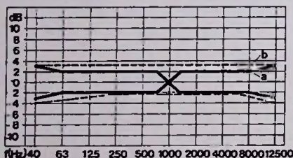
Bild 3. Toleranzfelder des Übertragungsbereichs für Plattenspieler (a) und Cassetten-Deck (b)
