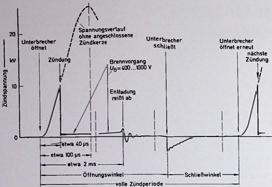
Bild 4. Spannungverläufe an der Zündspule während einer vollen Zündperiode
