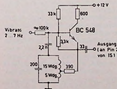
Bild 3. Stromlaufplan des 8-MHz-Oszillators
