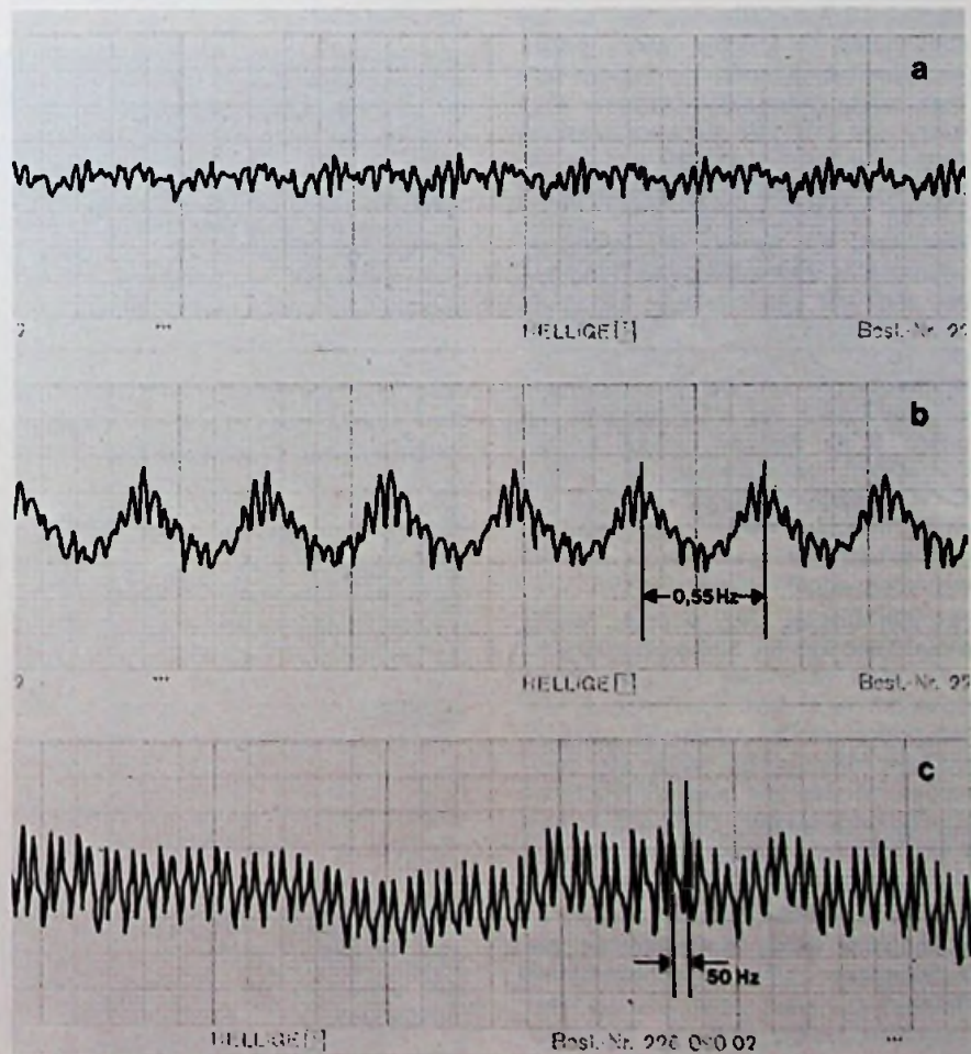
Bild 1. Gleichlaufmessungen an Plattenspielern mit dem Tonhöhenchwankungs-Messer EMT 420 A und dem Schnellschreiber Helcoscriptor HE 16. a) Gleichlauf eines Plattenspielers mit Zentralantrieb, b) Störeinfluß eines Schlages des Plattentellers je Umdrehung, c) Störeinfluß einer ellförmig laufenden Antriebsrolle
