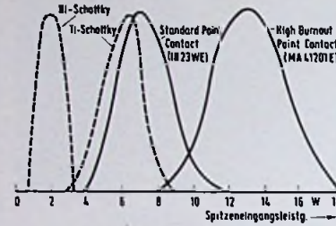
Bild 13. HF-Impuls-Burn-out für Si-Punkt-kontakt- und Schottky-Dioden. Pulsbreite 10 ns, 1000 Impulse/s, Frequenz 9,375 GHz, Rauschfaktorverschlechterung für Durchbruch = 1dB
