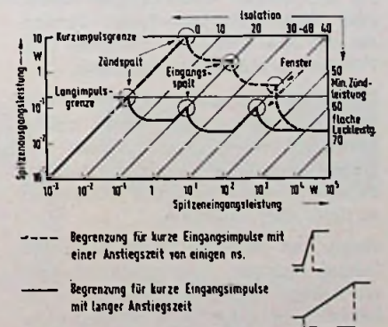
Bild 4. Typische Begrenzerlinie für den TR-Limiter (TRL)
