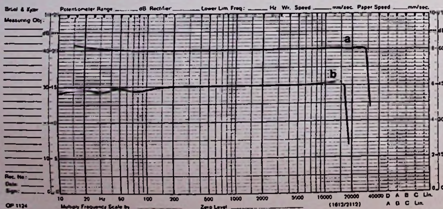
Bild 4. Typischer Frequenzgang eines Plattenspielers (a) und eines Cassetten-Decks (b)
