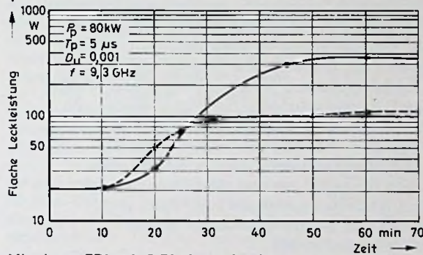
Bild 19. Verlauf der Konvektions- und künstlichen Kühlung
