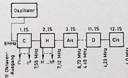
Bild 1. Übersichtsschaltplan des Generators mit zwölf integrierten Schaltungen
