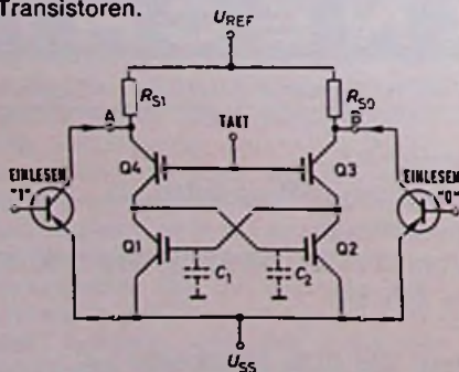
Bild 1. Schaltbild des RAM, Typ NEC 6002 (Nortec)
